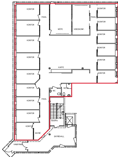
UTSNITT NORR, PLAN 1
